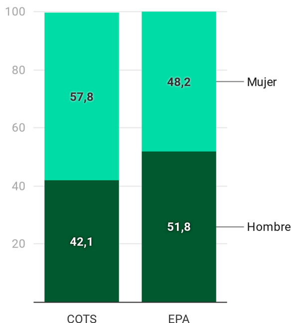
Figura 3. Género COTS/EPA
